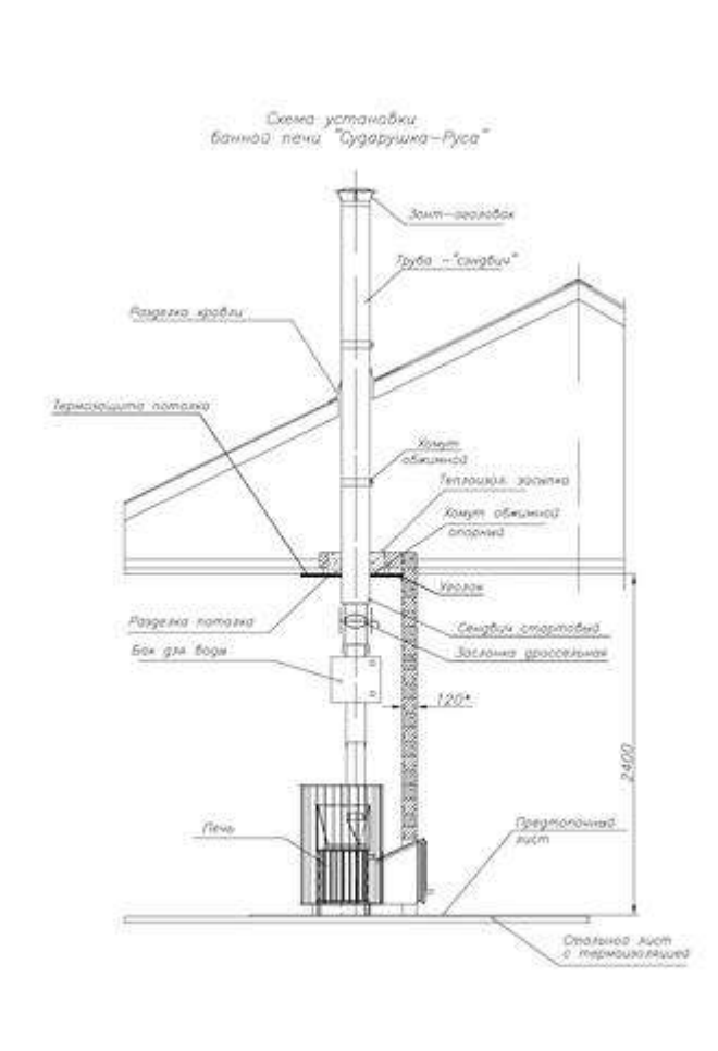
Рис. 4. Схема установки печи
