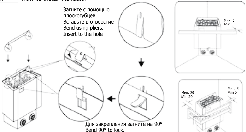
Рис. 2 | Установка теплоотражателя Fig. 2 | How to install Reflector
