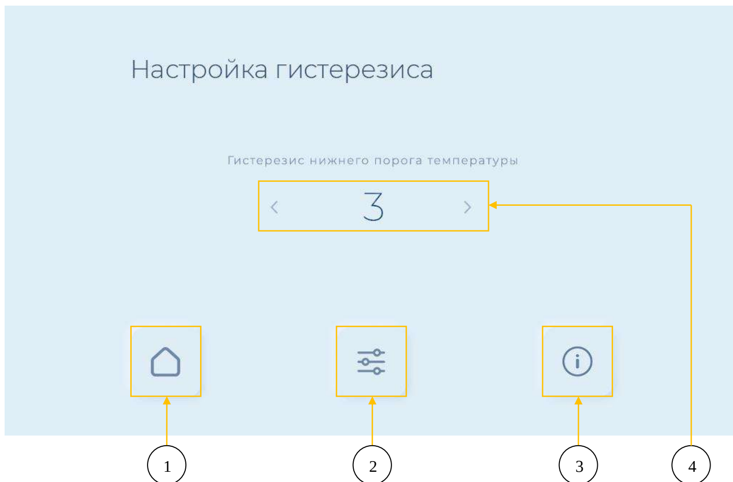
Рис. 36. Взаимное расположение элементов интерфейса страницы “настройка гистерезиса”
