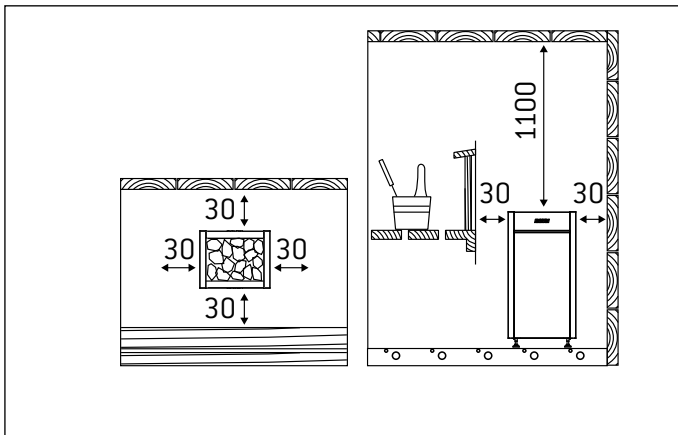
Рисунок 5. Расстояния безопасности (все размеры приведены в миллиметрах) Joonis 5. Kerise miinimum ohutuskaugused (kõik mõõdud millimeetrites)
