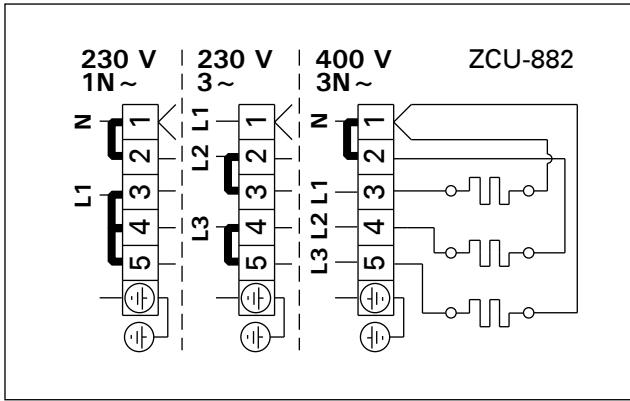
Рисунок 9. Электромонтаж Joonis 9. Elektri hendused
