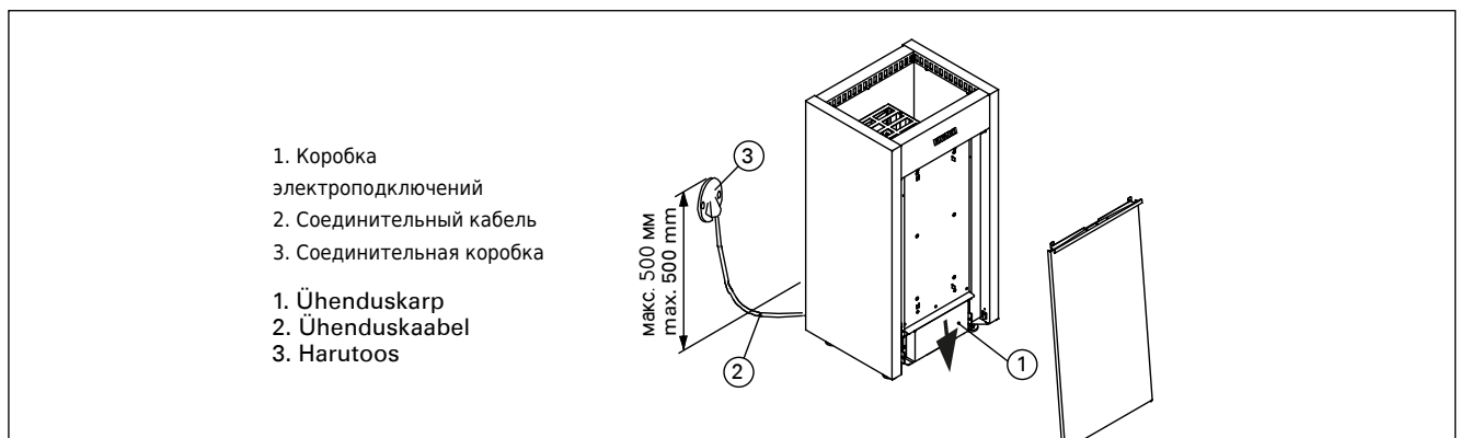
Рисунок 7. Установка каменки Joonis 7. Kerise ühendamine elektrivõrgu
