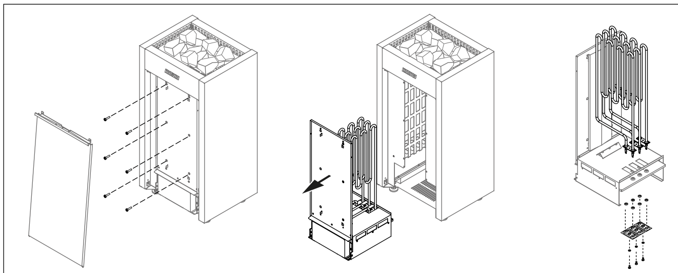
Рисунок 8. Замена нагревательных элементов Joonis 8. K ttelementide vahetamine
