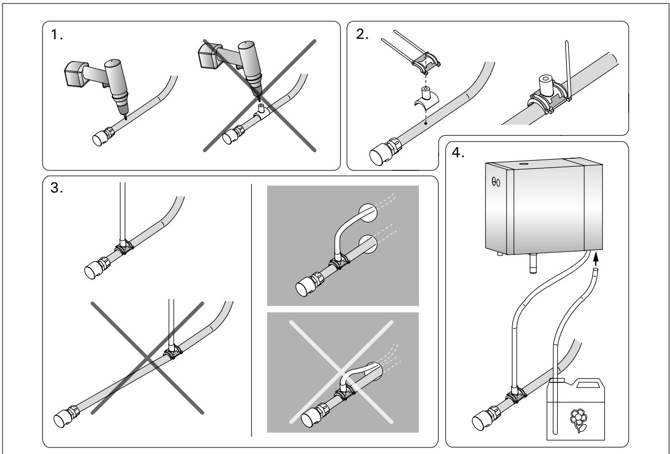
Рисунок 11. Подключение устройства подачи ароматизатора Joonis 11. L hnaaine pumba toru paigaldamine
