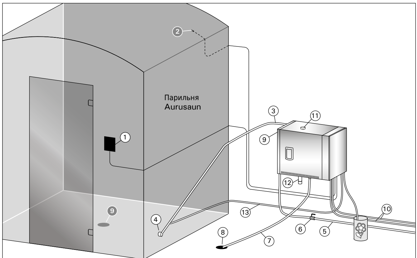
Рисунок 1. Элементы системы парогенератора Joonis 1. Aurugeneraatori s steemi komponendid
