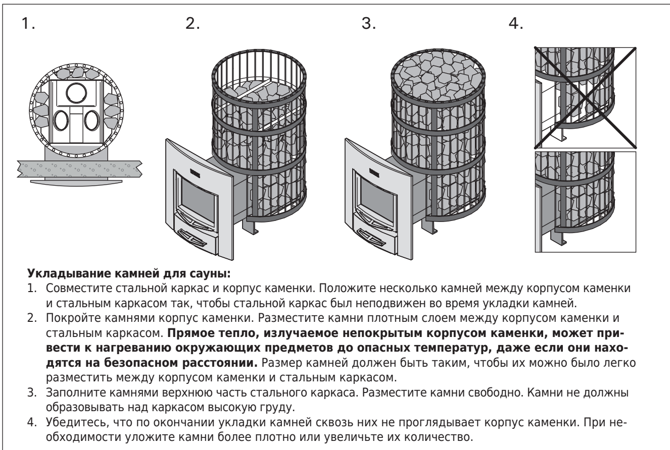
Рисунок 3. Укладка камней
