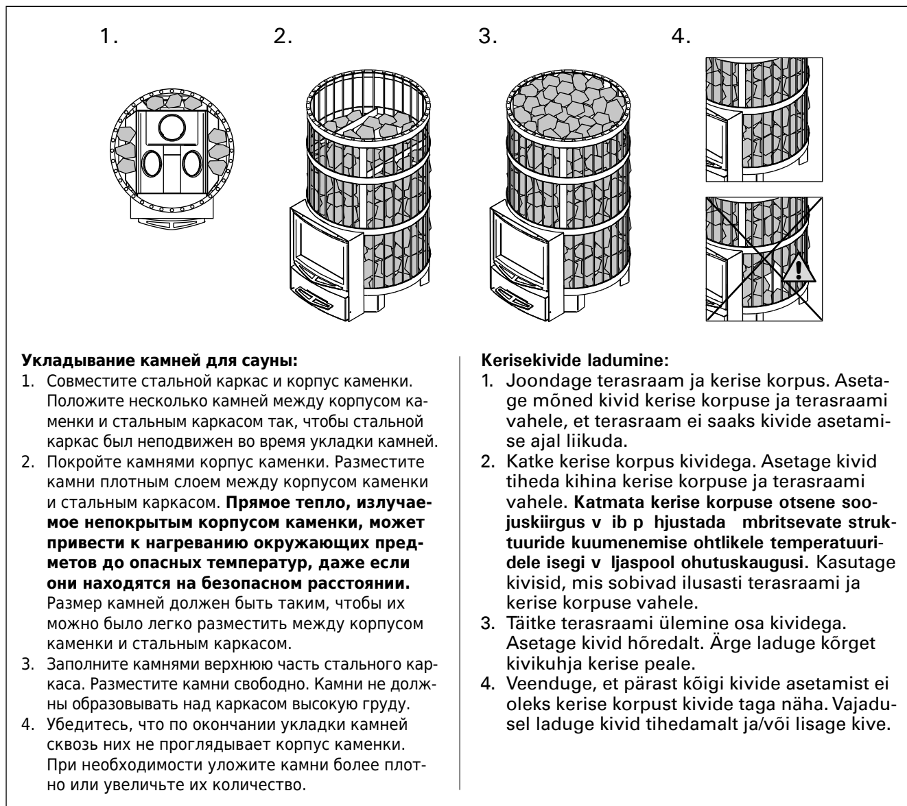
Рисунок 3. Укладка камней
