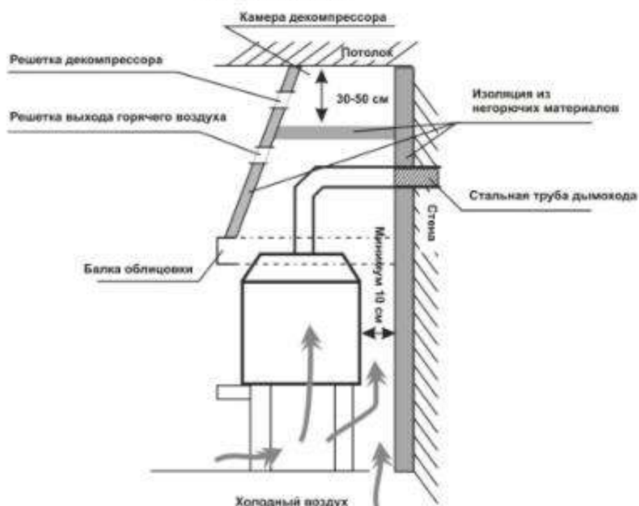
РИСУНОК 4: ВИД СБОКУ
