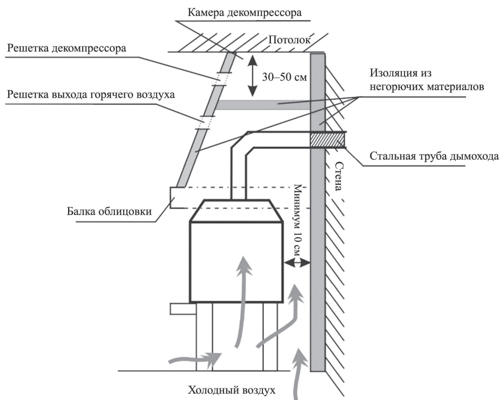
Рис. 4. Вид сбоку
