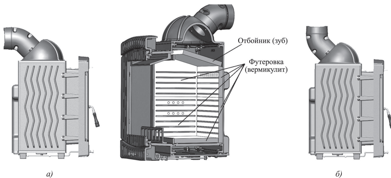
Футеровка.
